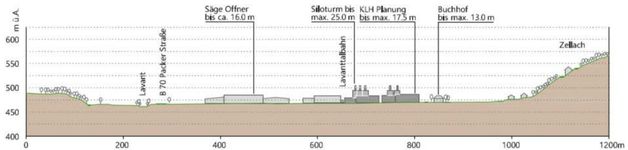
Schemaschnitt in Südost-Nordwest-Richtung von Frantschach blickend
