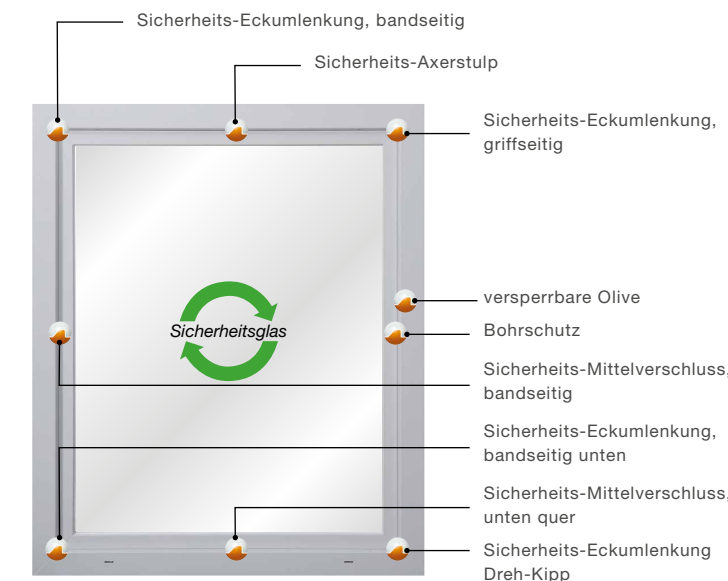
EINBRUCHSICHERHEITS-KLASSE RC3 Das AluFusion Fenstersystem Contur 95 erhalten Sie in der Einbruchsicherheitsklasse RC3. Dies garantiert Ihnen Sicherheit auf höchstem Niveau.
