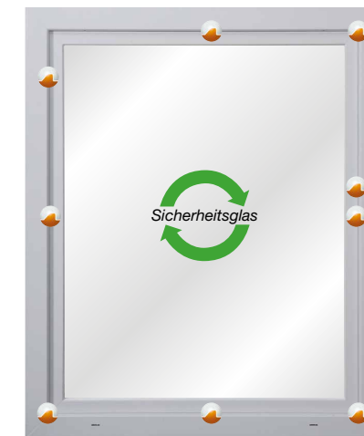
EINBRUCHSICHERHEITS-KLASSE RC2 (optional) Verriegelung mit Pilzpfenverschlüssen, zusätzliche Ausstattung mit Sicherheitsglas und versperrbarer Olive
