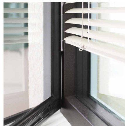
INTEGRIERTE JALOUSIEN bestechen, zwischen den Fensterscheiben montiert, besonders mit ihrem geringen Pflegeaufwand und der dezenten Optik. Bei der cleveren Systemlösung RUPO-AddOn ist diese praktische Jalousien-Variante bereits serienmäßig integriert.
