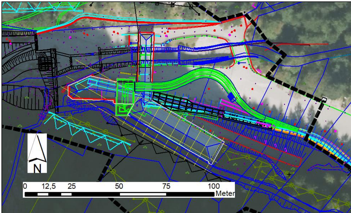
Abbildung 3: Lageplan Herren-Rodelstart (grün) (Quelle: Deyle 2026) über Luftbild
