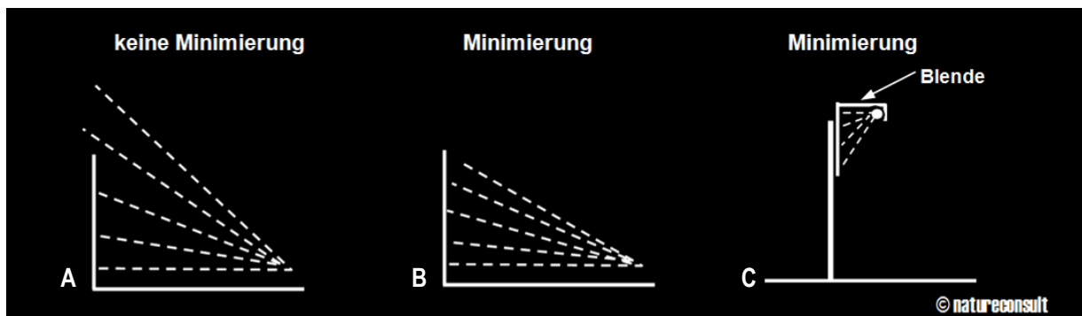
Abbildung 20: minimalinvasive Verwendung von Beleuchtungseinrichtungen für Hinweisschilder an Wänden (A, B) und freistehende Hinweisschilder (C) (verändert nach BCT & ILE 2005)
