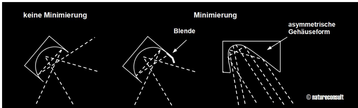
Abbildung 22: minimalinvasive Verwendung von Beleuchtungseinrichtungen durch gerichtete Abstrahlwinkel bzw. Blenden (verändert nach BCT & ILE 2005)
