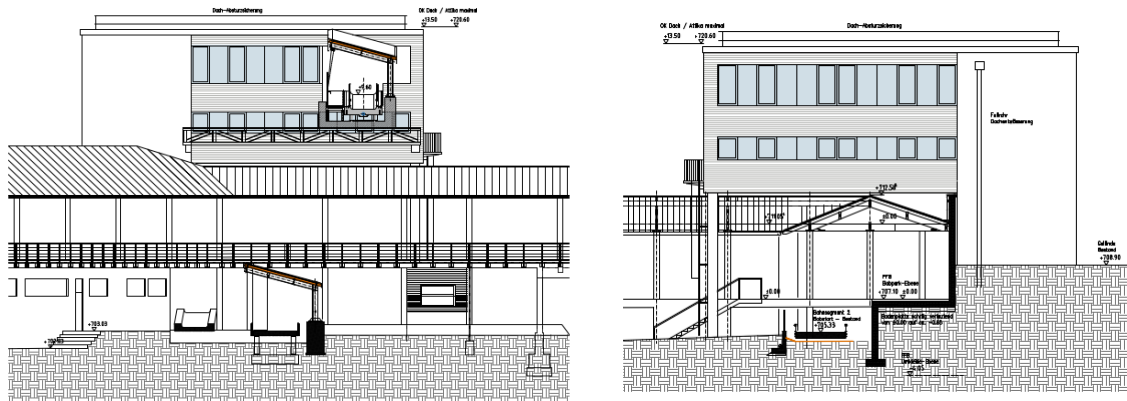
Abbildung 5: Ansicht Herrenrodelstart von Osten (links) und Westen (rechts) (Quelle: Deyle 2026)
