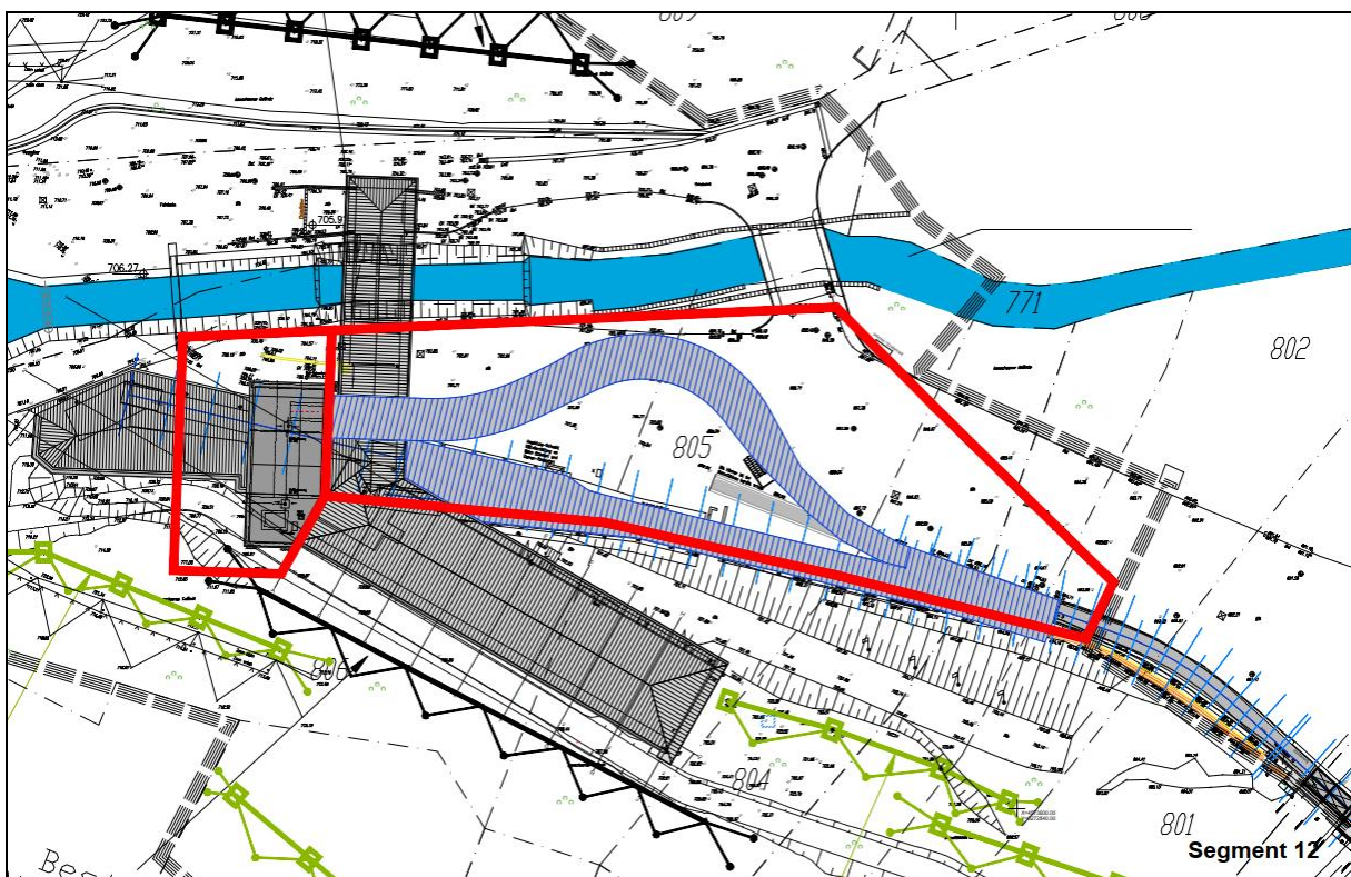
Abbildung 2: Lageplan Abgrenzung Planungsbereich gemäß Vereinbarung mit BUND (Quelle: Deyle 2026)
