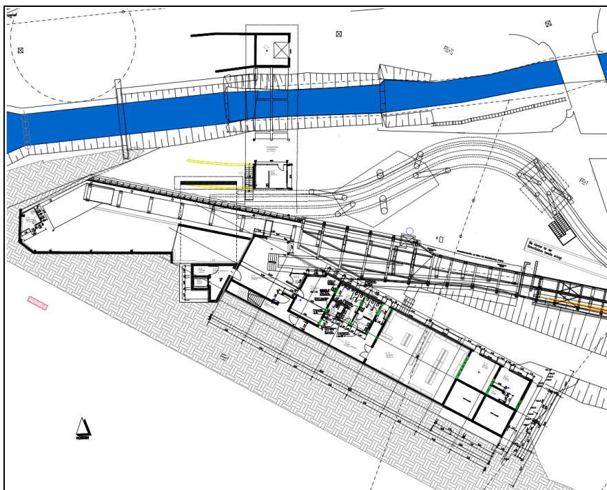
Abbildung 4: Neuausrichtung Herren-Rodelstart – Grundriss UG (Quelle: Deyle 2026)
