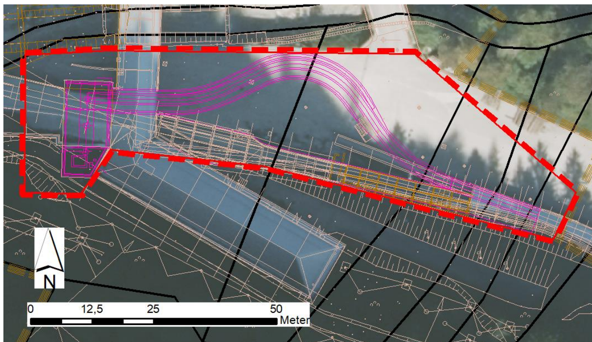
Abbildung 18: Lageplan Neuausrichtung Herrenrodelstart mit Neuansbindung an Bestandsbahn (pink) mit Bearbeitungsgebiet (rot) über Luftbild (Befliegung 21.09.2024)
