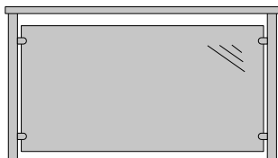
Basismodell Glasfüllung ohne Rahmen Max. Steherabstand 1400 mm!
