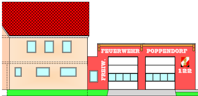
GEPLANTER ZUBAU ANSICHT VON LANDESSTRASSE
