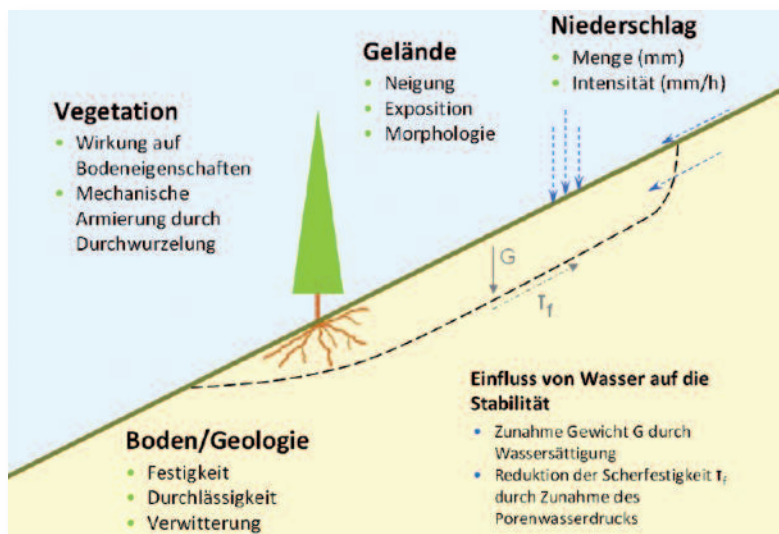
Abbildung 1: Einfluss verschiedener Faktoren auf die Hangstabilität (Rickli, 2001) [6]
