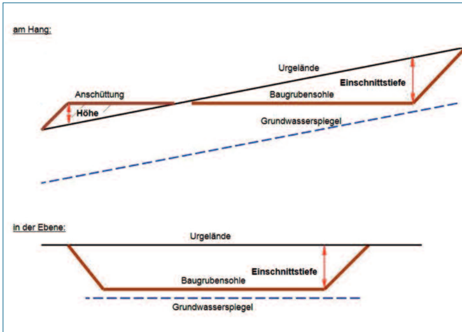
Abbildung 4: Höhenbezüge bei Einschnitten und Aufschüttungen
