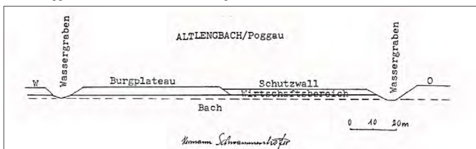
Abb.3: Lageschnitt von H.Schwammenhöfer
