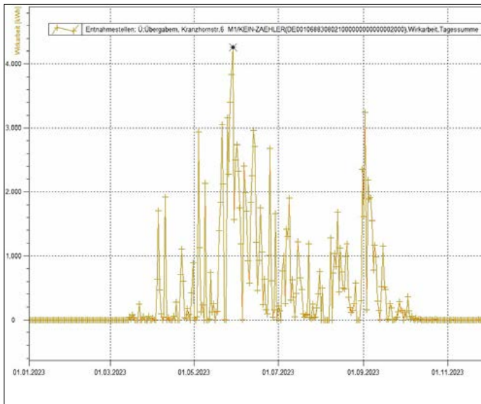
Netzurückspeisung
