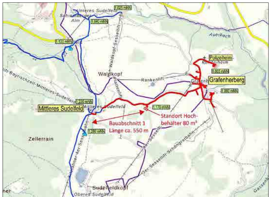
Neue Trinkwasserversorgung Grafenherberg Bauabschnitt I
