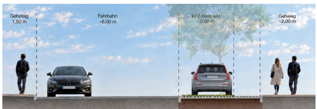
Querschnitt Ungarnstraße neu Grafik: beigestellt/Stadtgemeinde Fehring
