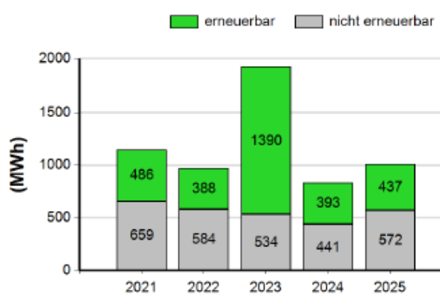
Anteil erneuerbarer Wärme
