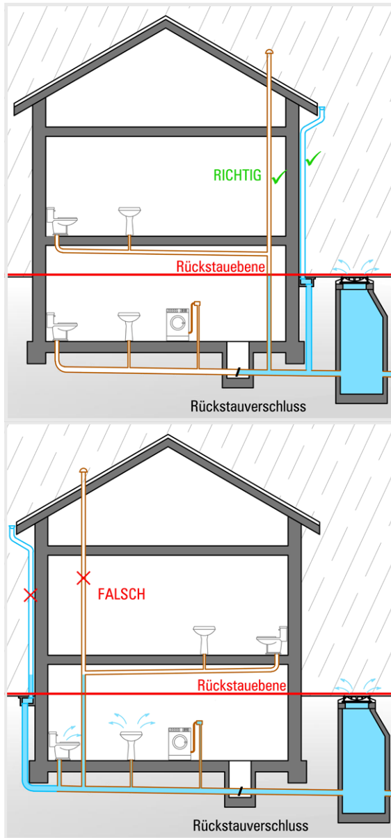
Abbildung 8 | Rückstauverschluss - richtige und falsche Anordnung
