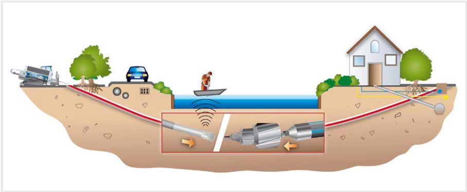
Abbildung 16 | Prinzipskizze Spülbohrung
