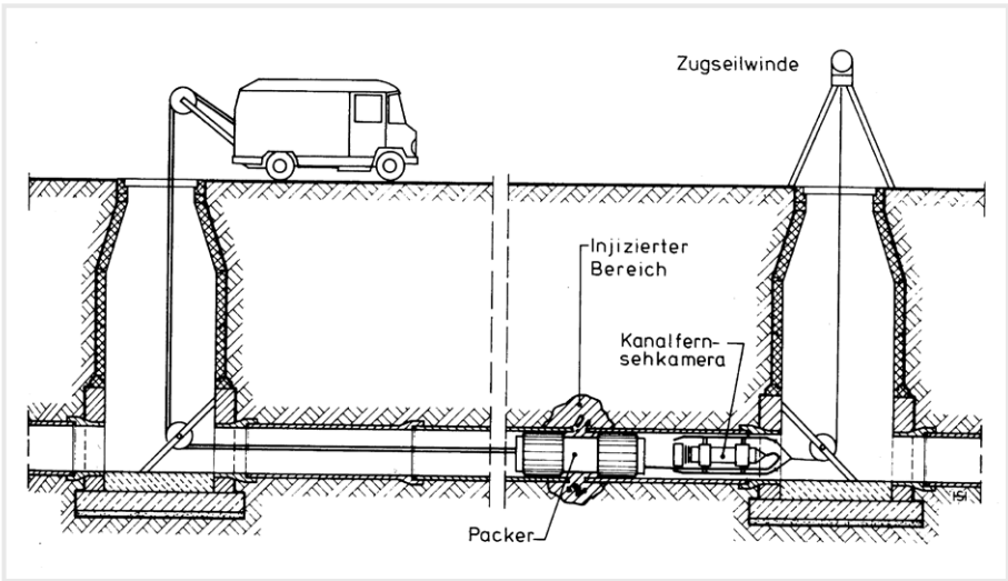
Abbildung 33 | Prinzipskizze Packerverfahren
