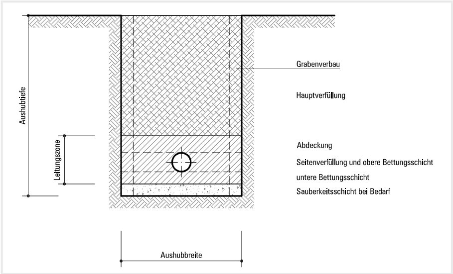
Abbildung 13 | Querschnitt Kanalkünette
