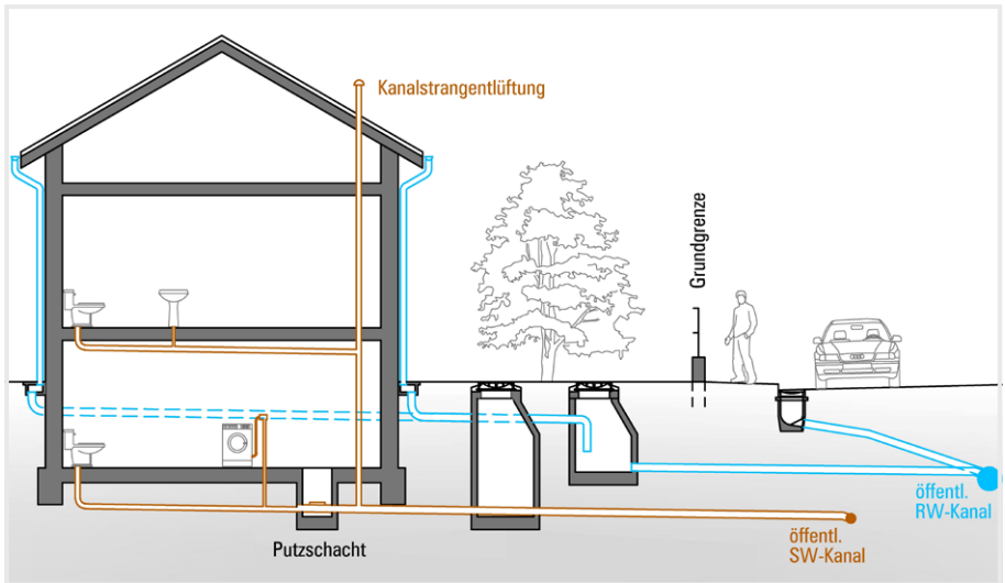
Abbildung 9 | Trennsystem
