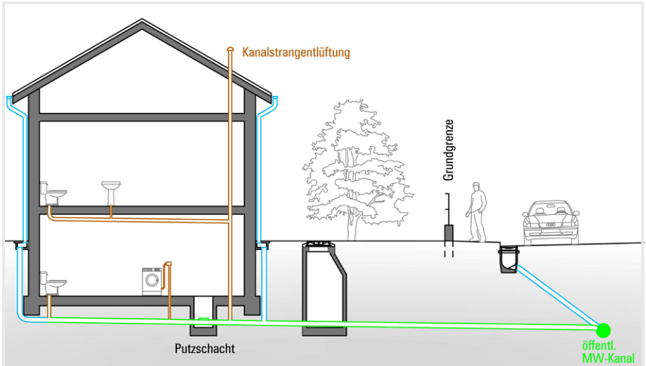
Abbildung 10 | Mischsystem
