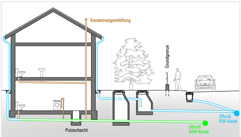
Abbildung 11 | Qualifiziertes Mischsystem
