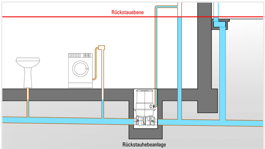
Abbildung 7 | Rückstauhebeanlage
