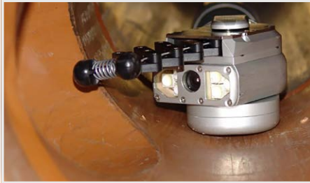
Abbildung 30 | Satellitenkamera im Hauskanal
