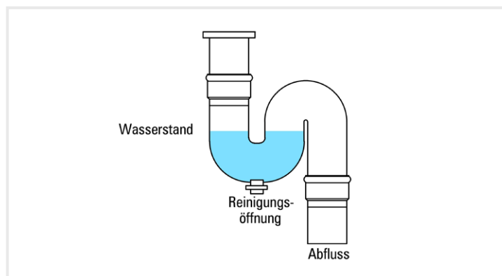
Abbildung 3 | Geruchsverschluss
