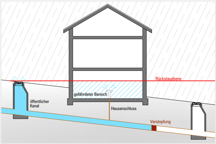
Abbildung 5 | Rückstauenebene, maßgebliche
