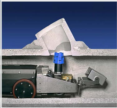
Abbildung 31 | Robotersanierung
