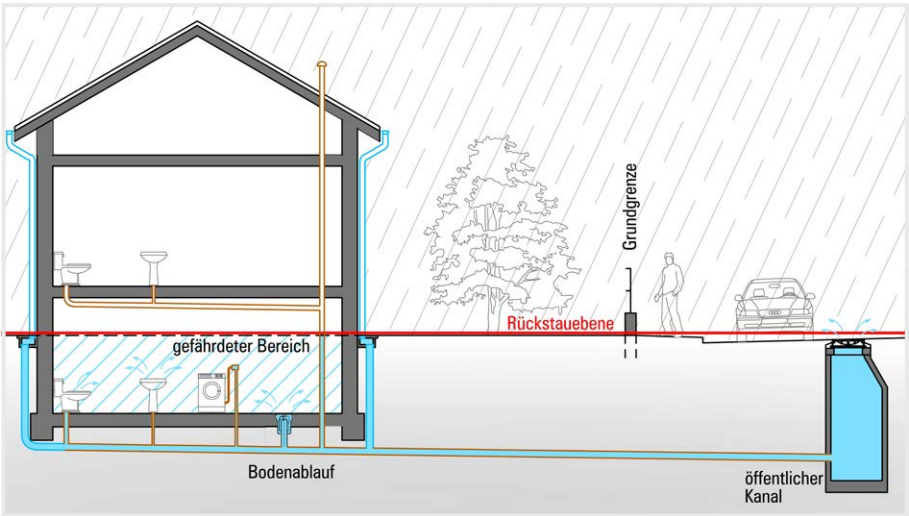
Abbildung 6 | Rückstauenebene, maßgebliche
