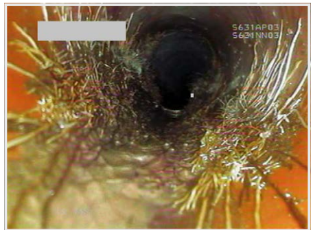
Abbildung 23 | Durchwurzelung
