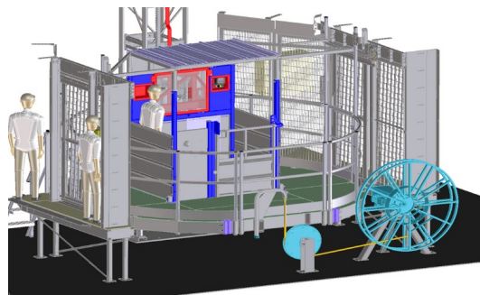
„Gittermastbühne“
