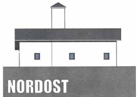
Teilansichten des Feuerwehrhauses nach Um- und Zubau aus dem Einreichplan
