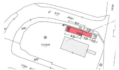
Planansicht des neuen Bauhof-Schutzdachs
