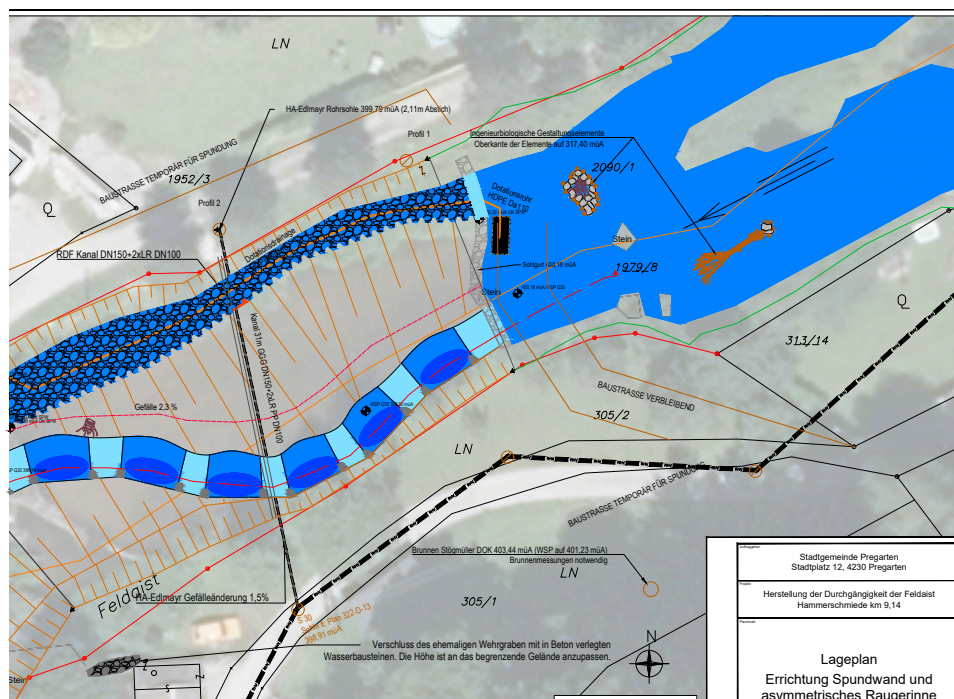
Staubeereich der Hammerschmiede bei Kilometer 9,14 | Grafik: Wasser und Land Ziviltechniker GmbH
