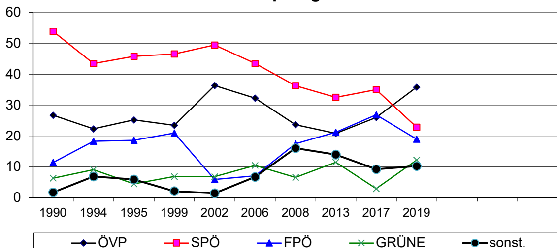
Nationalrat: Prozentanteile Sprengel 3 1990 - 2019
