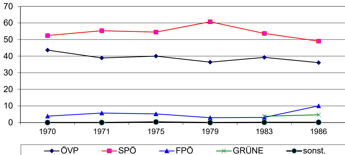
Nationalrat: Prozentanteile Sprengel 3 1970 - 1986
