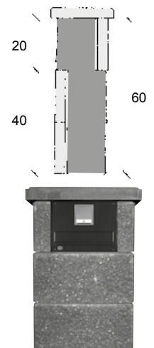
Briefkasten mit Einwurfklappe
