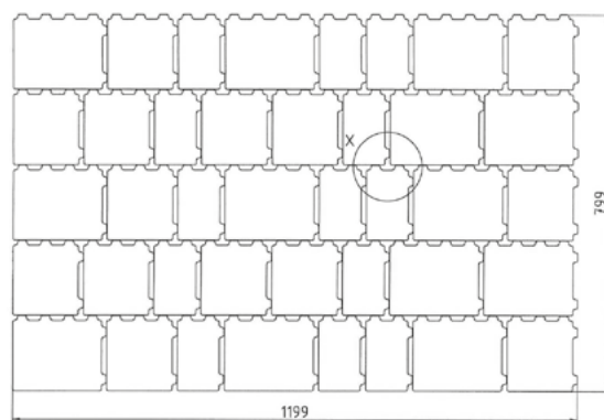
ÖKO - INNOVO mit Sickerfuge
