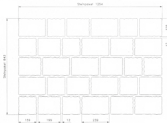
Santino Pflasterlage
