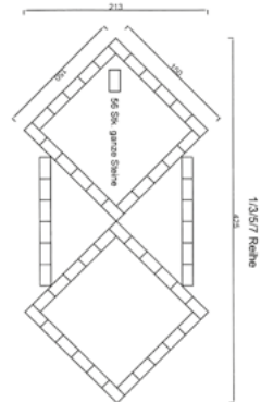
Hochbeet Palma
