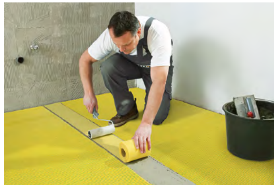
Verlegung über alten Bestand: Fliesen, Holz, Beton
