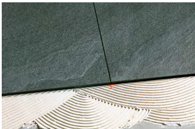
Verlegung in Klebemörtel
