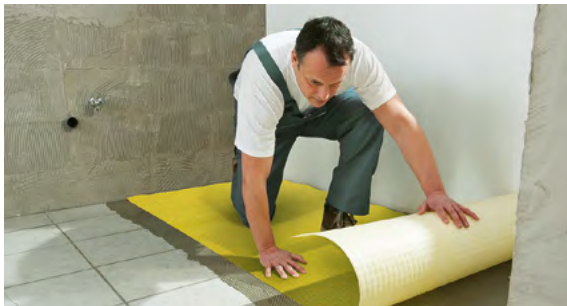
Verlegung über alten Bestand: Fliesen, Holz, Beton
