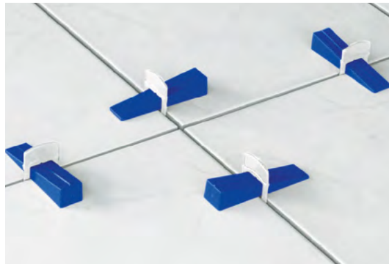
Keil und Lasche für Nivelliersystem
